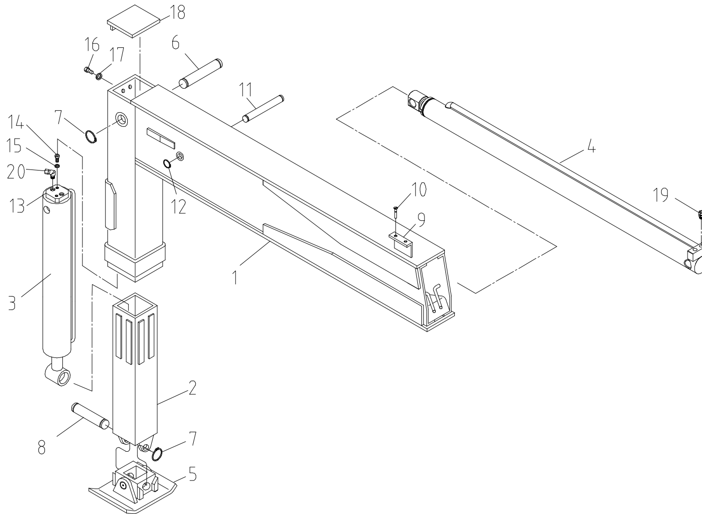
아우트리거 조립체(8톤) Fig. 4 SCS746L OUTRIGGER ASS'Y(8TON)
