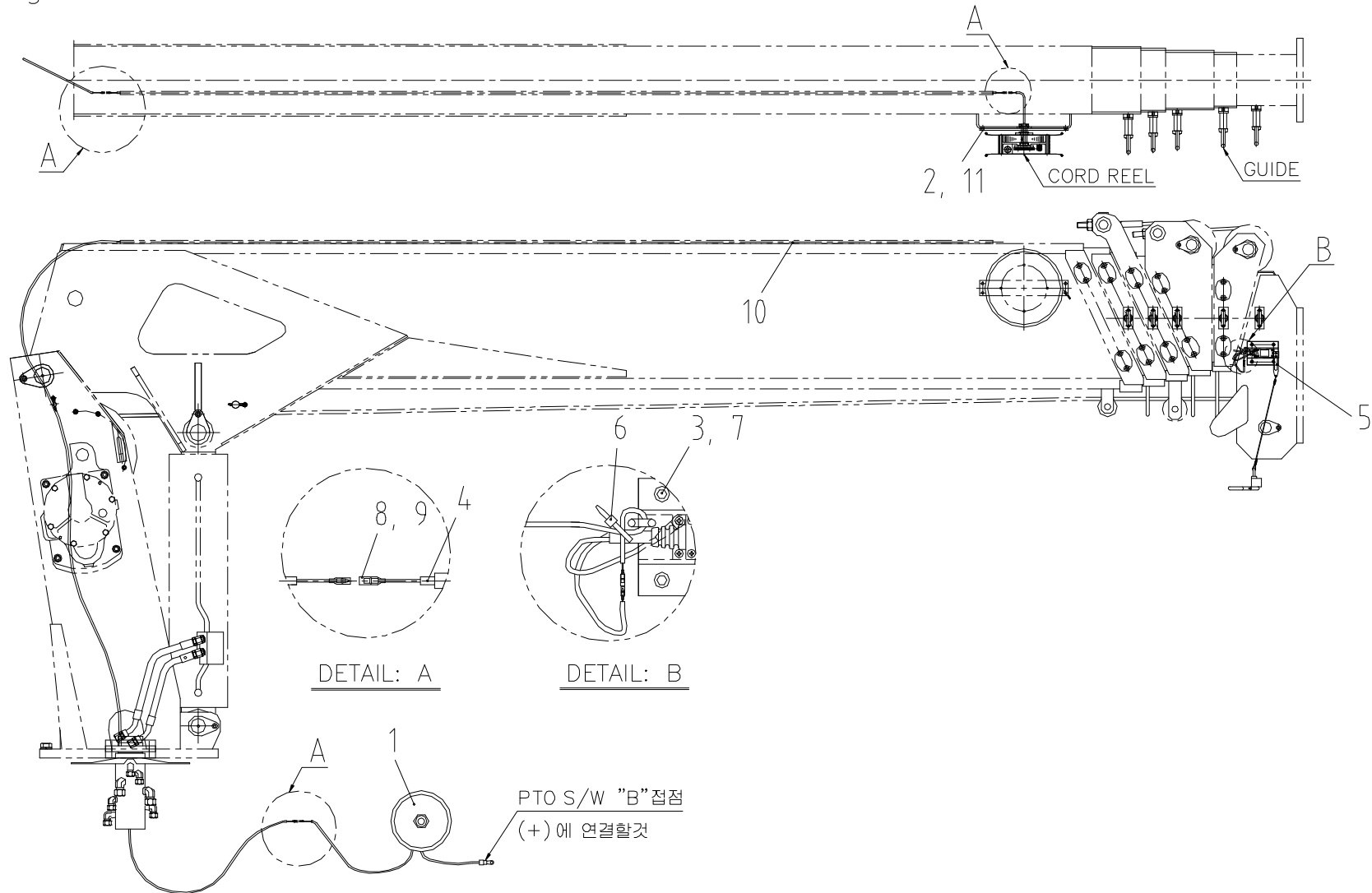
Fig. 13 과권방지장치 조립체
