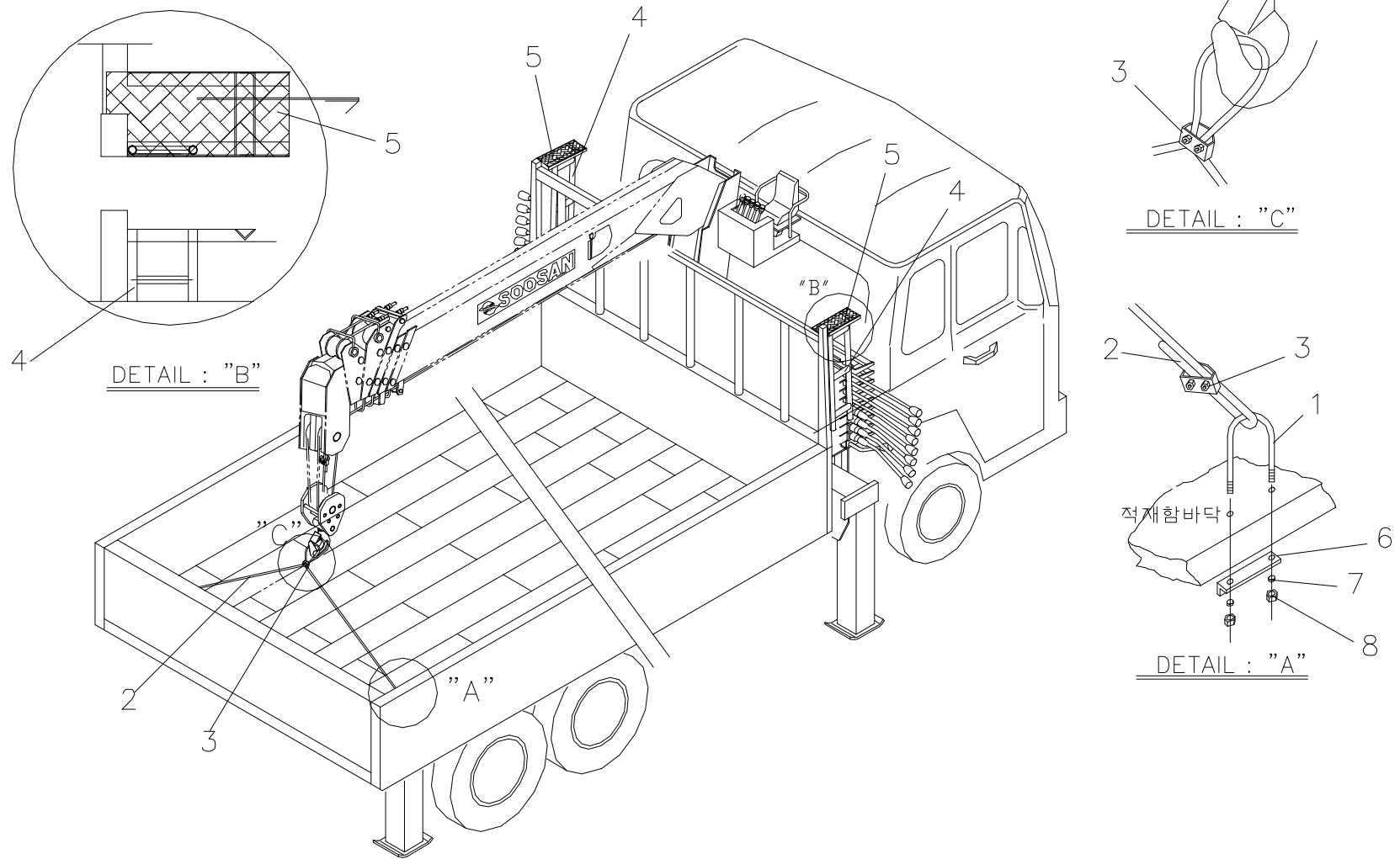
로딩 박스 파트 Fig. 8-5 SCS746L LOADING BOX PART
