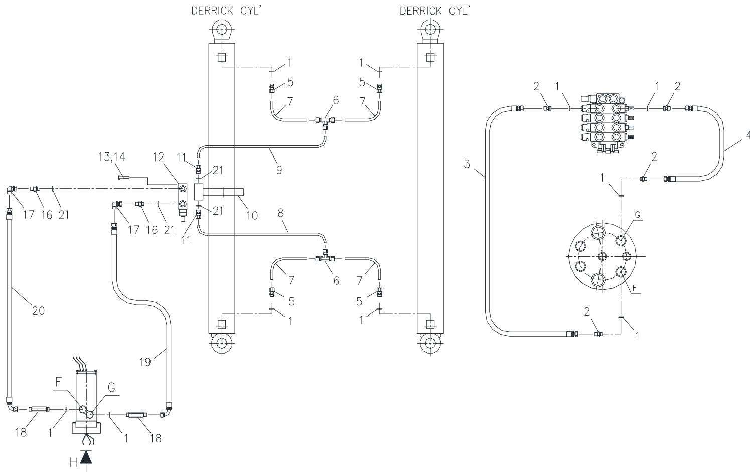
데릭 배관 (표준형) Fig. 5-2 SCS746L DERRICK PIPING (STD)
